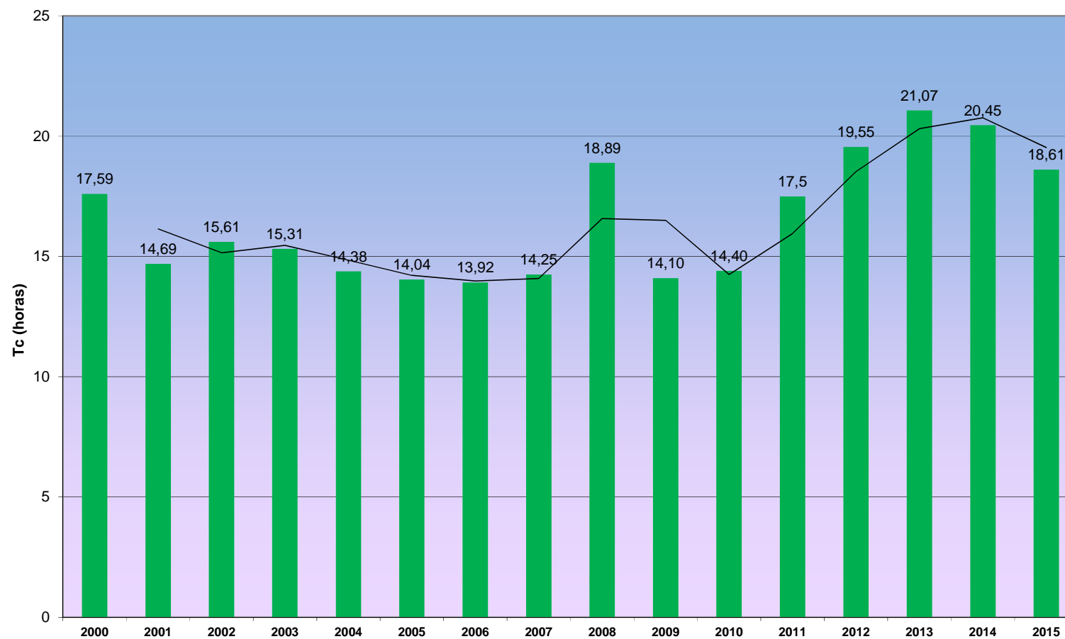
GRAFICO 12: EVOLUCION MEDIA CIER Tc (horas)
