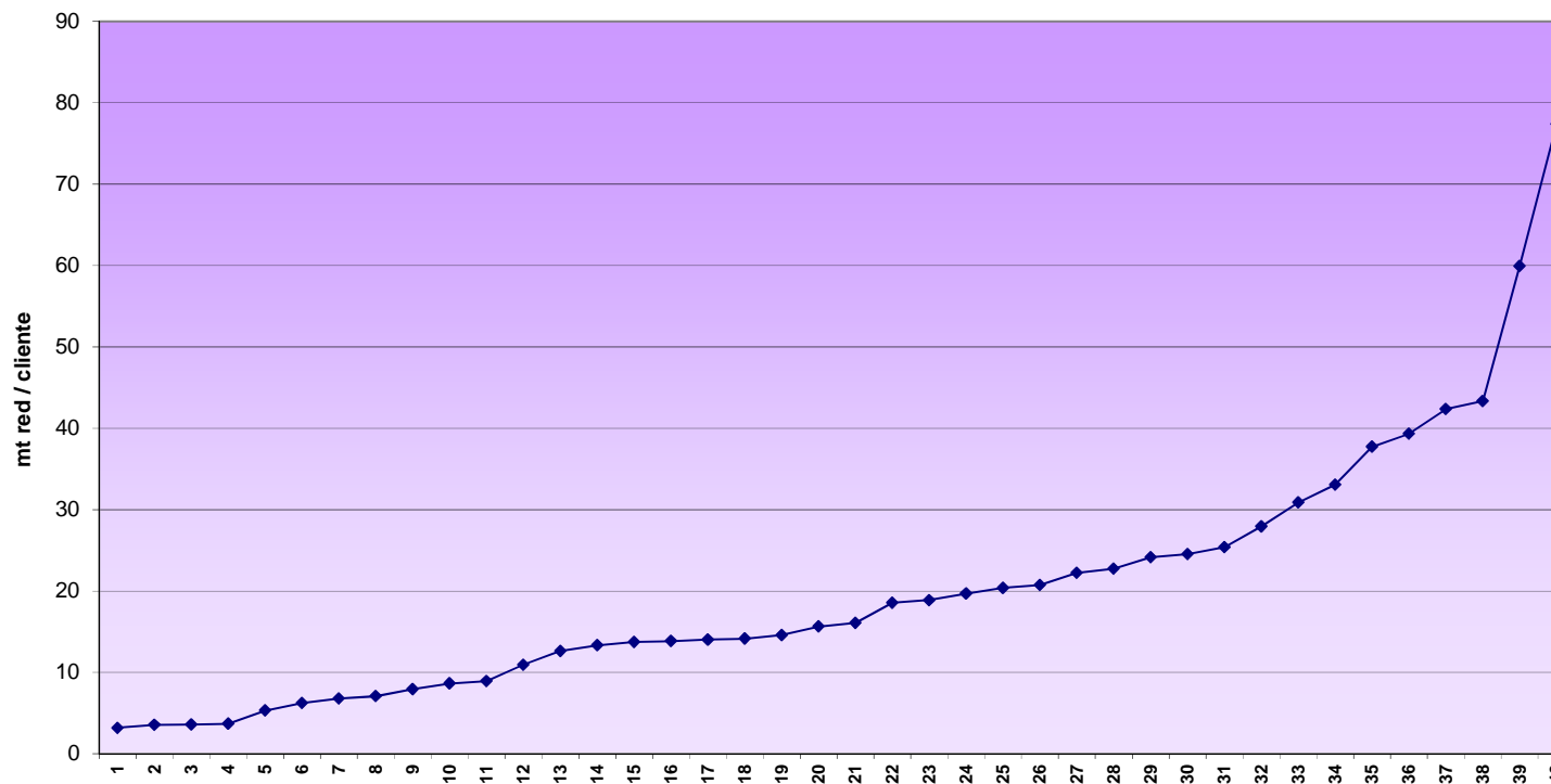
GRAFICO 7: EXTENSION DE RED DE MT POR CLIENTE – (METROS DE RED DE MT/CLIENTE)
