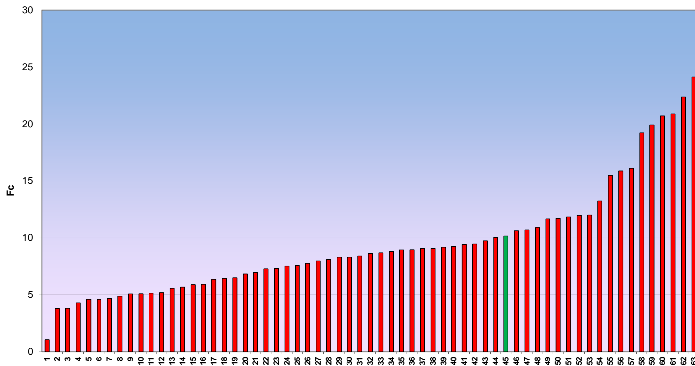
GRAFICO 1: FRECUENCIA MEDIA DE INTERRUPCIÓN POR CLIENTE (Fc)
