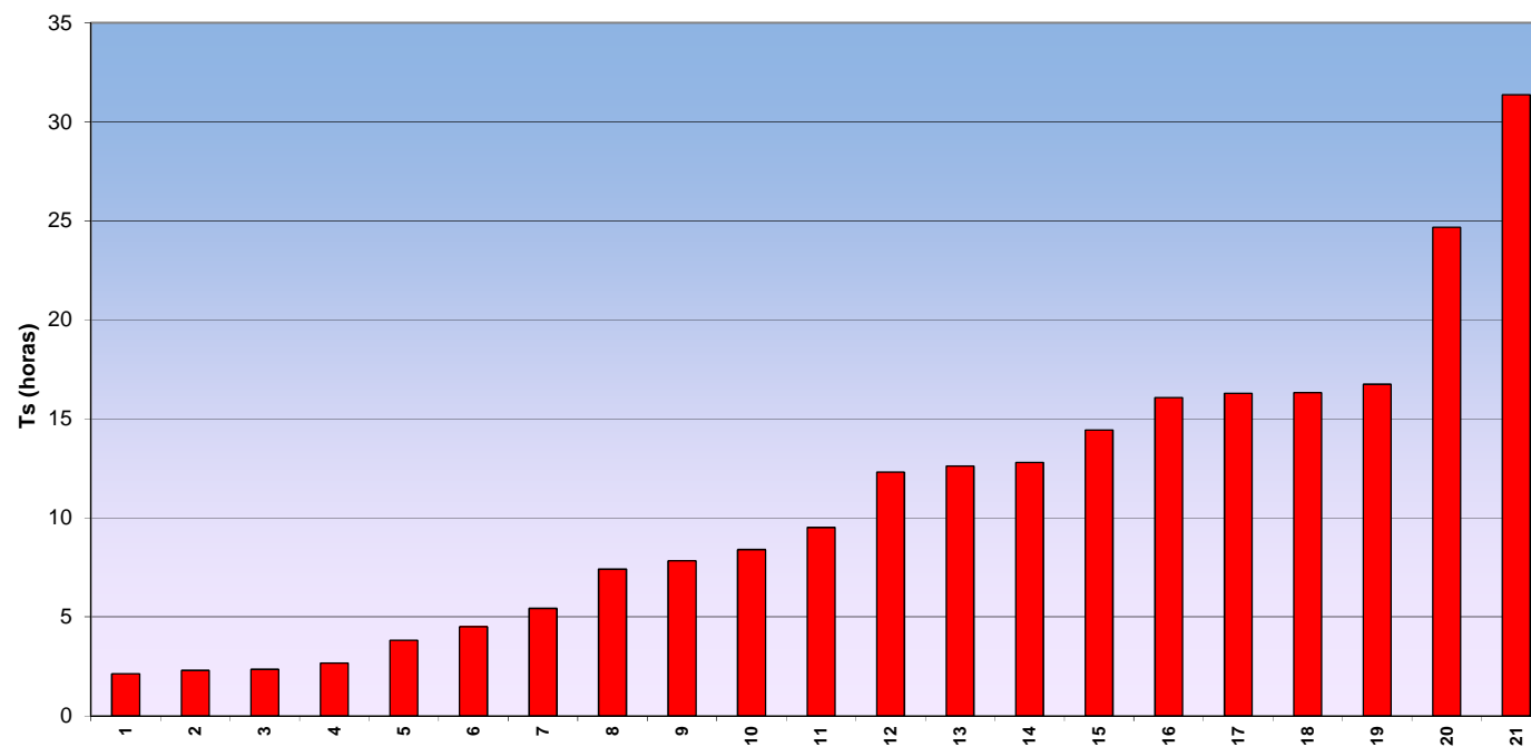
GRAFICO 5: TIEMPO TOTAL DE INTERRUPCIÓN POR POTENCIA (Ts horas)
