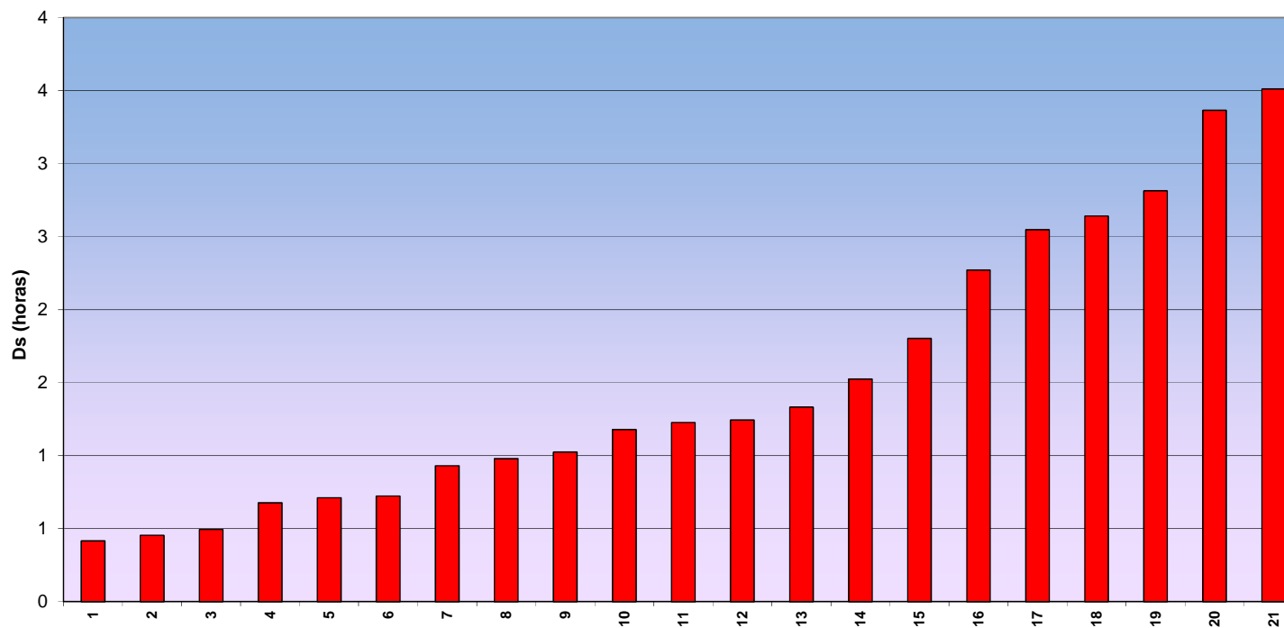
GRAFICO 6: DURACIÓN MEDIA DE LAS INTERRUPCIONES-POTENCIA (Ds horas)
