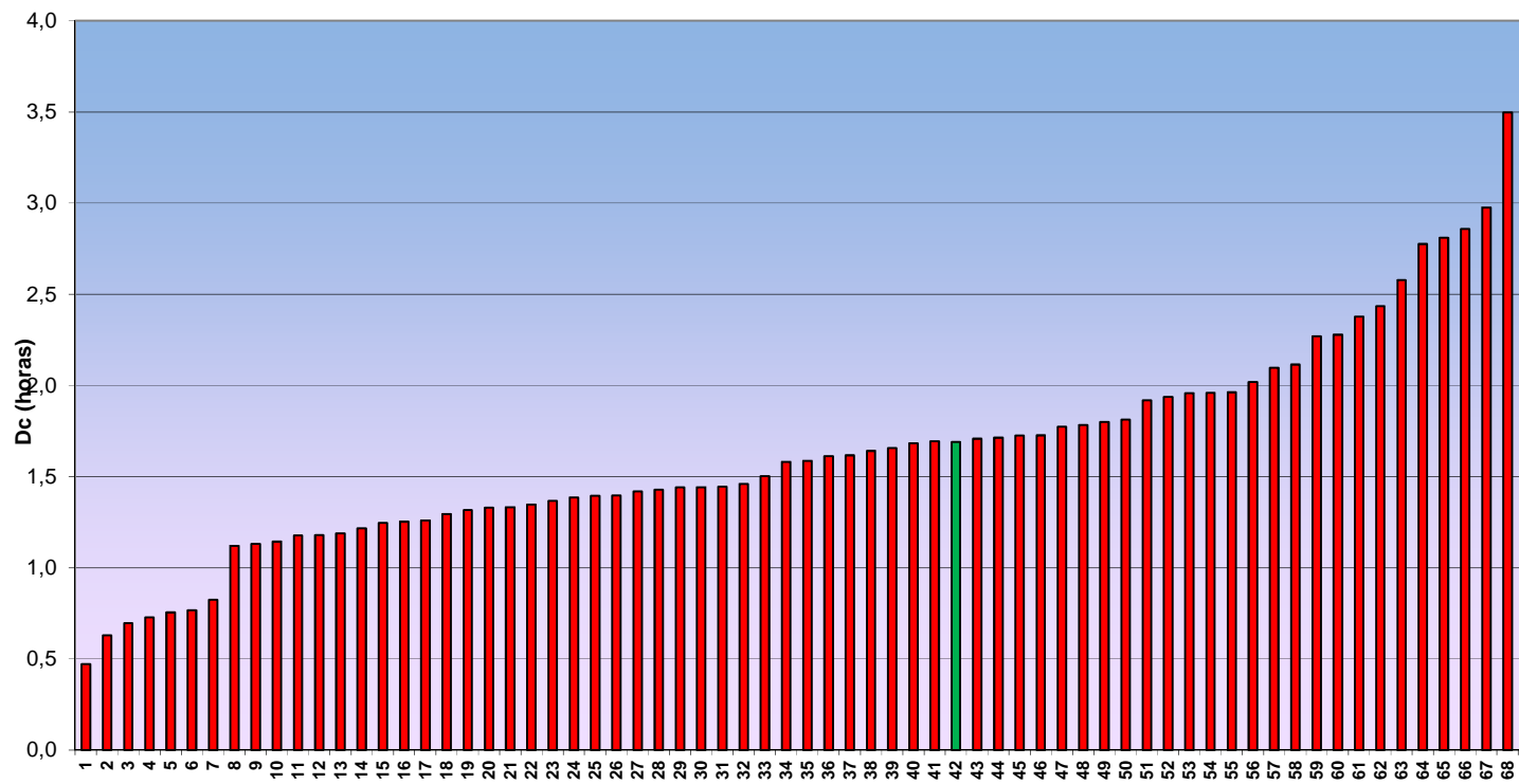
GRAFICO 3: DURACIÓN MEDIA DE LAS INTERRUPCIONES-CLIENTE (Dc horas)
