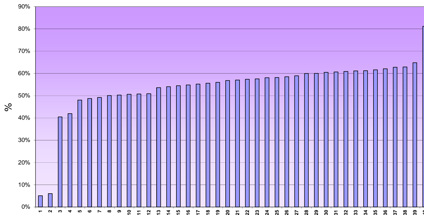
GRAFICO 8: % ENERGIA / POTENCIA PICO * 8760 HORAS AÑO
